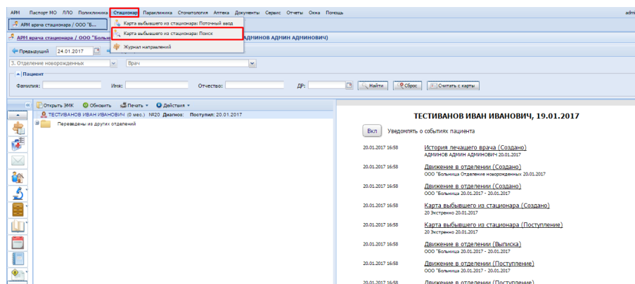
Рис. 2: Поиск КВС
